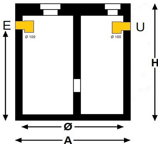
SEZIONE VERTICALE
