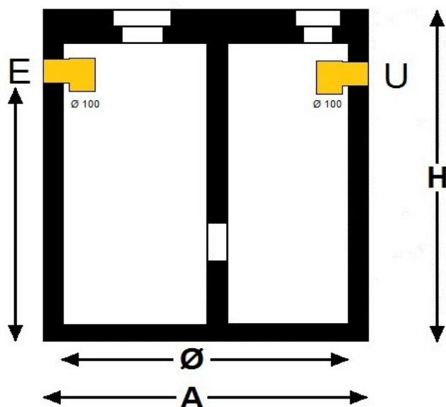
SEZIONE VERTICALE
